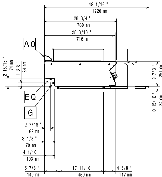
Oldalnézet
